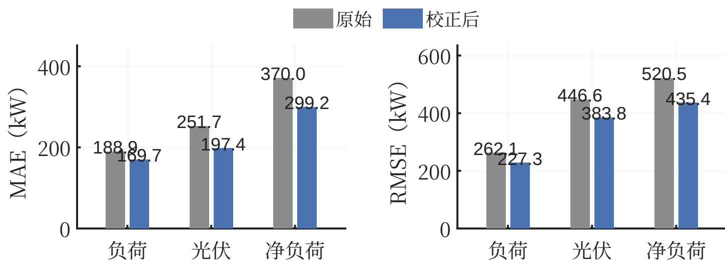
偏差校正前后的预测误差：MAE 与 RMSE
